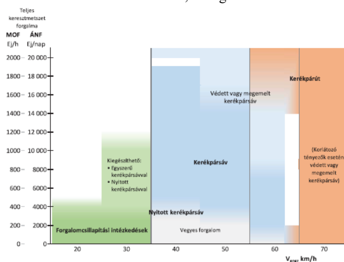
1. ábra. Kerékpárosbarát kialakítás minimális kiépítési szintjei a tervezett gépjárműforgalom és a tervezett engedélyezett sebesség függvényében lakott területen.
