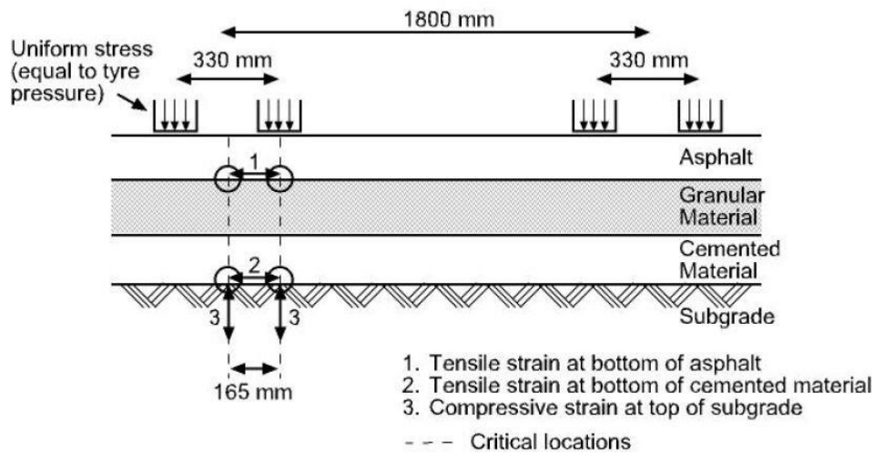
1. ábra: Pályaszerkezeti modell, (Austroads, 2012)
