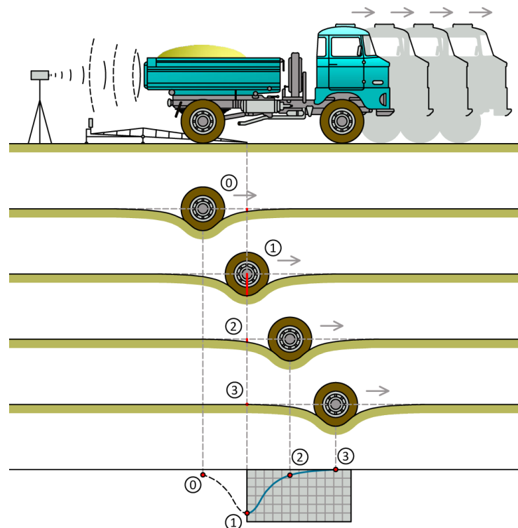
2. ábra: A továbbfejlesztett kézi behajlásmérés elve
